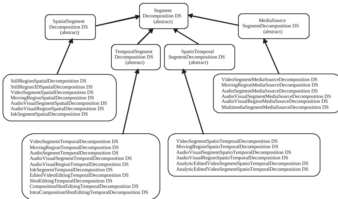
FIG. 2.5 – Hiérarchie des différentes décompositions structurales applicables aux segments
