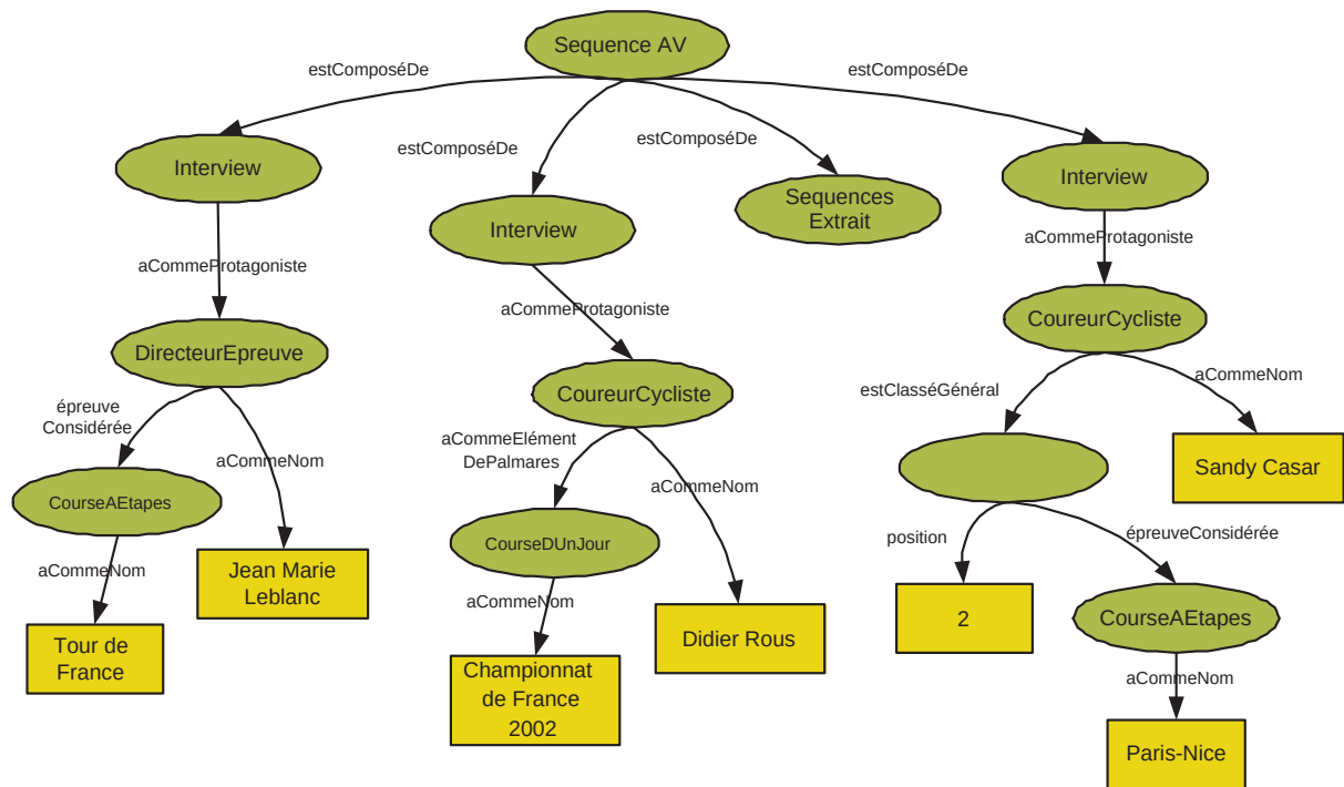
FIG. 4.2 – Description sémantique de la séquence numérotée 12 du tableau 4.1 sous la forme d'un graphe RDF
