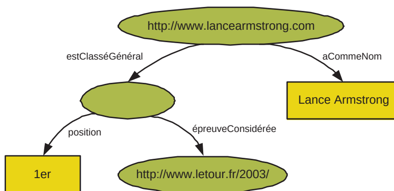
FIG. 3.5 – Exemple de graphe RDF représentant l'assertion du tableau 3.1
