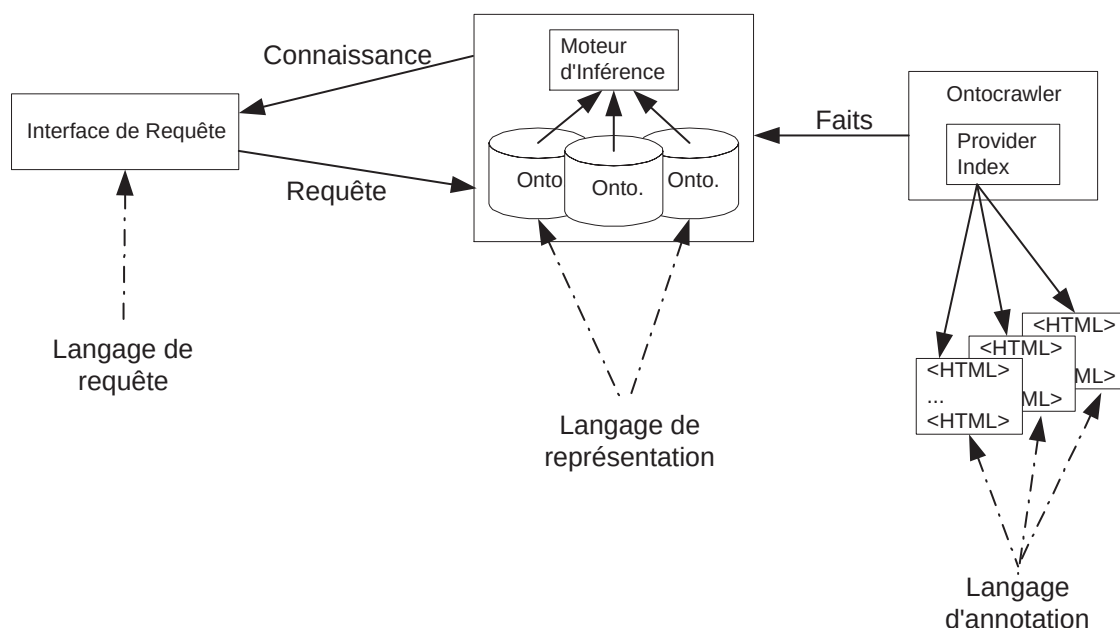
FIG. 3.4 – Architecture générale d'Ontobroker
