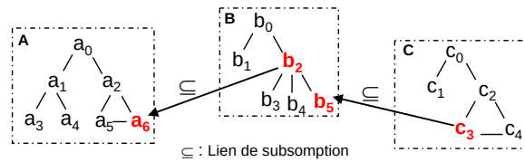
Fig.2 – Ajout de correspondances par composition.
