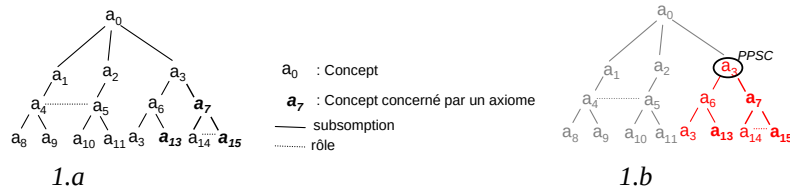
FIG. 1 – Segmentation d'une ontologie.
