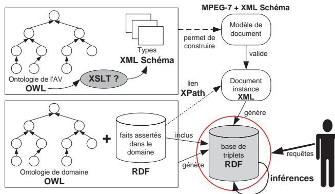
FIG. 4 – Proposition d'architecture pour permettre le raisonnement dans les descriptions documentaires. L'ontologie de l'AV permet de formaliser les connaissances structurales des descriptions. Elle est traduite en types XML Schema pour pouvoir exprimer des modèles de document et est instanciée lors de la description. Enfin, une autre ontologie de domaine, avec les faits qui y sont raccordés, permet d'exprimer la connaissance conceptuelle qui sera liée aux éléments structurels de la description.
